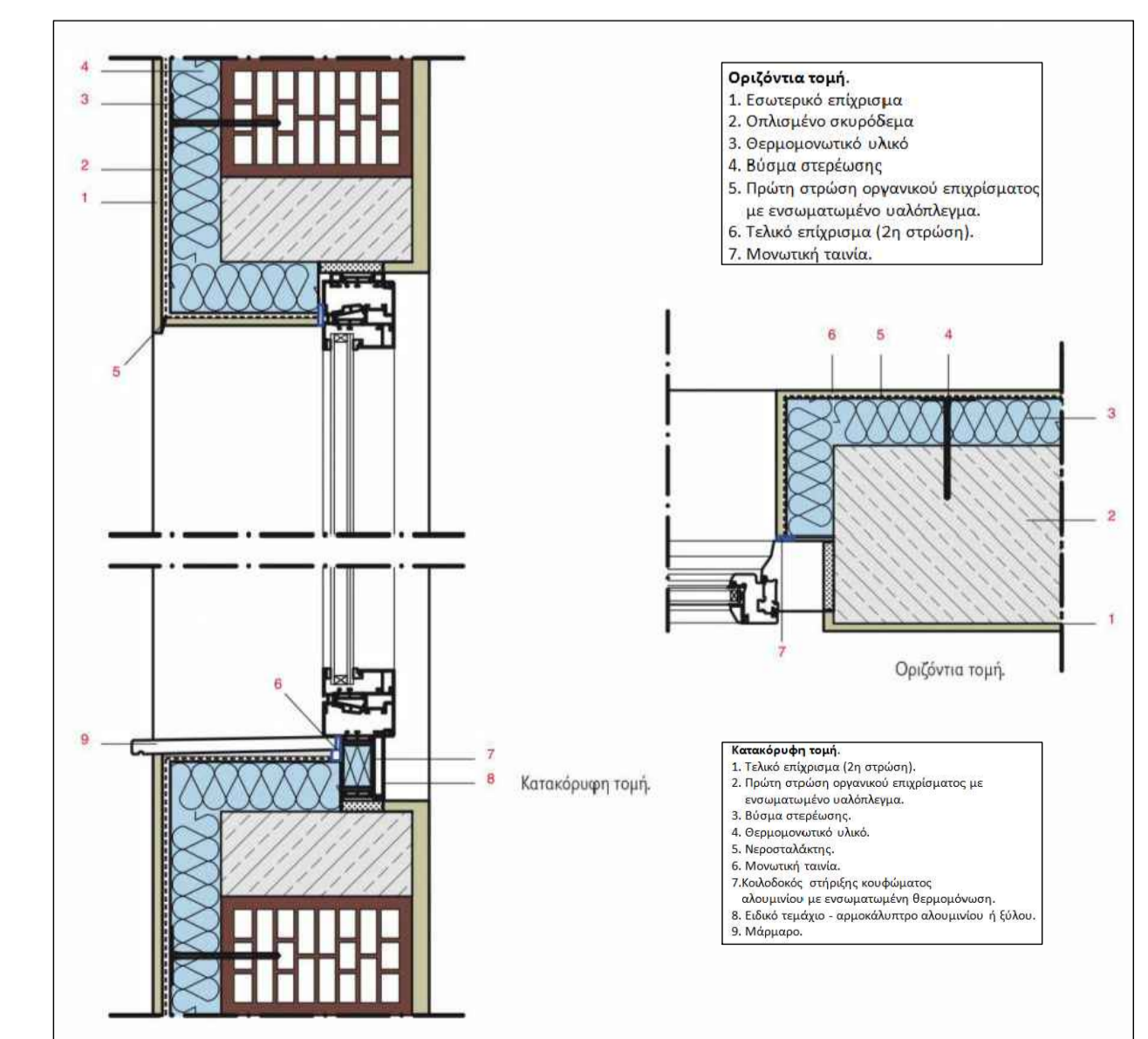
ΛΕΠΤΟΜΕΡΕΙΑ ΕΣΩΤΕΡΙΚΗΣ ΘΕΡΜΟΜΟΝΩΣΗΣ ΚΑΙ ΣΥΝΑΡΜΟΓΗΣ ΠΑΡΑΦΥΡΟΥ
