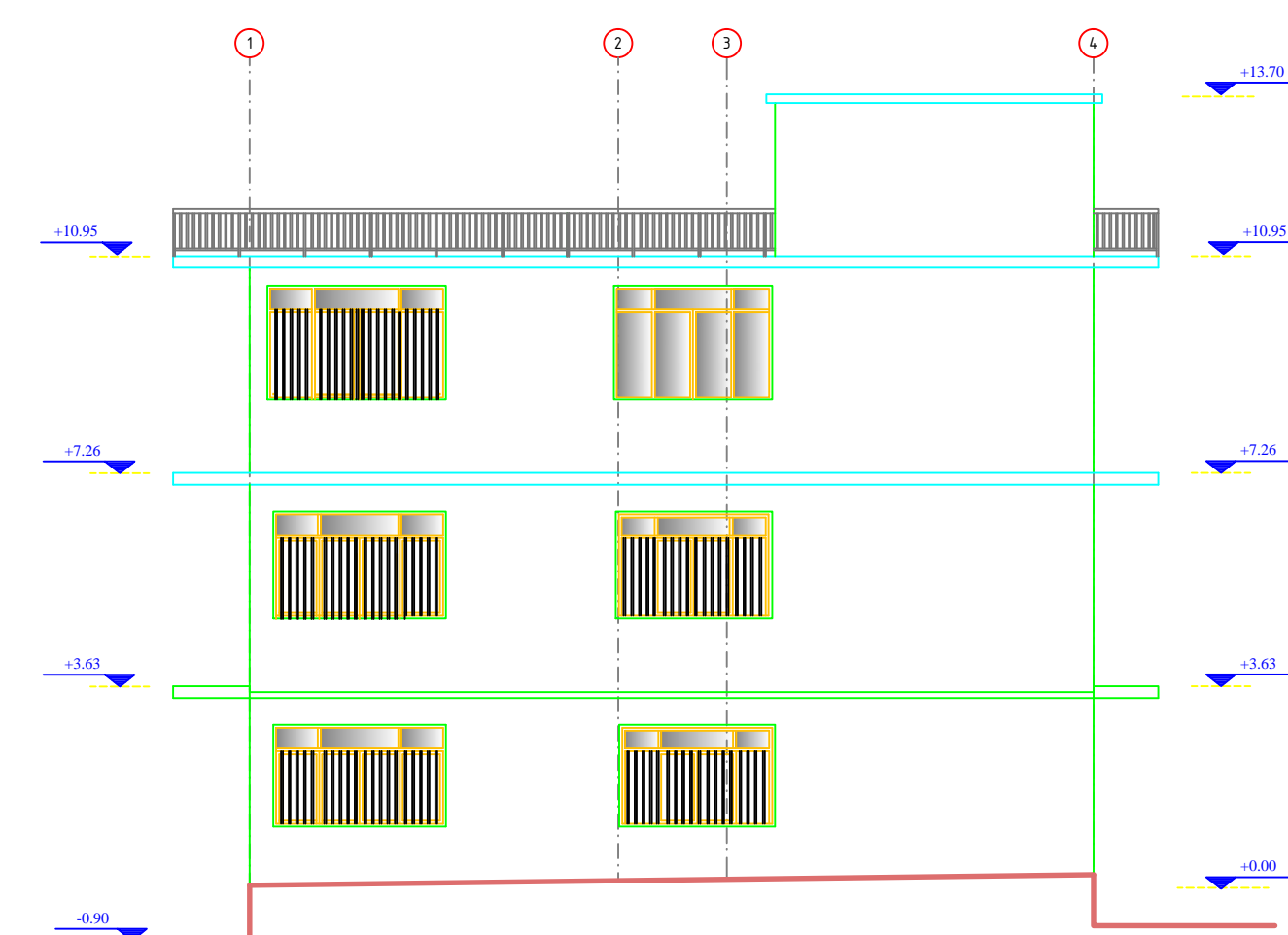
ΟΨΗ Α
