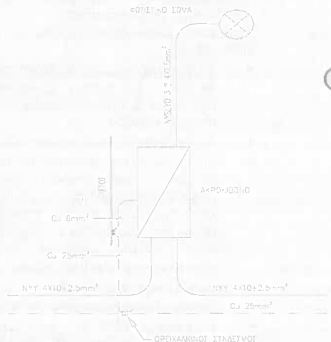
ΔΙΑΓΡΑΜΜΑ ΣΤΗΝΔΕΣΜΟΛΟΓΙΑΣ ΦΩΤΙΣΤΙΚΟΥ
