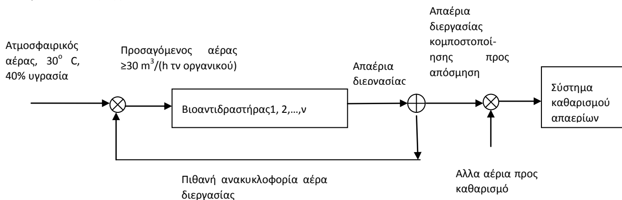
Σχήμα 1. Λειτουργία βιοαντιδραστήρων και συστήματος απόσπησης.
