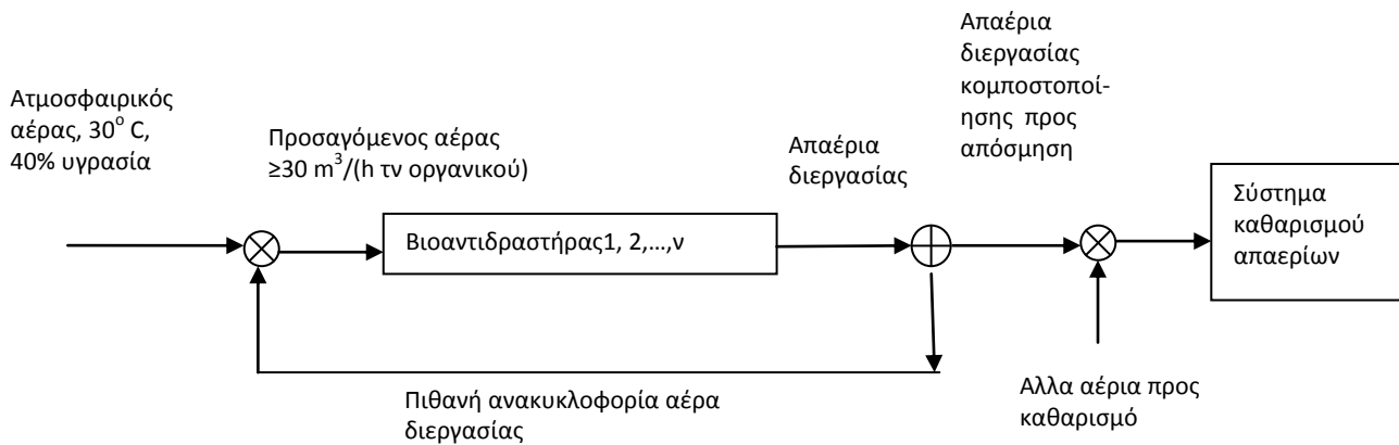
Σχήμα 1. Λειτουργία βιοαντιδραστήρων και συστήματος απόσμισης.
